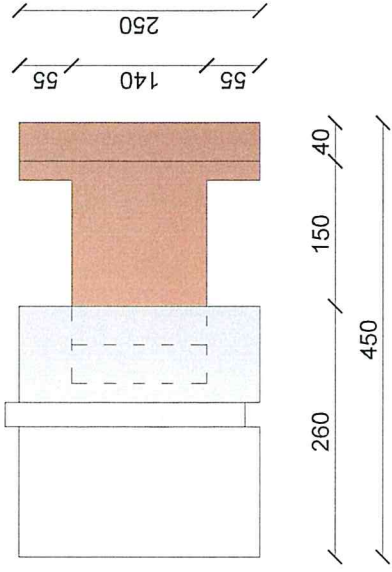
VISTA INTERNA
