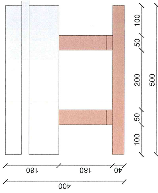
VISTA SUPERIORE
