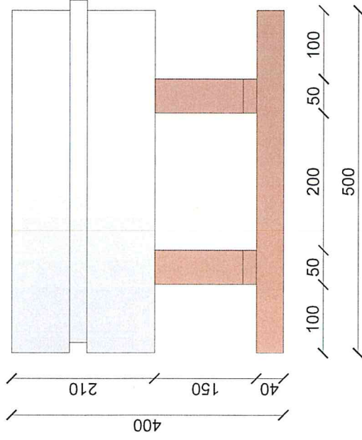
VISTA SUPERIORE
