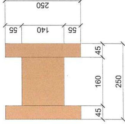
VISTA LATERALE
