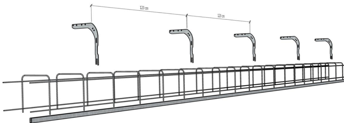
Figure 23 - Equerres de renfort (tous les 120 cm) et renfort en U
