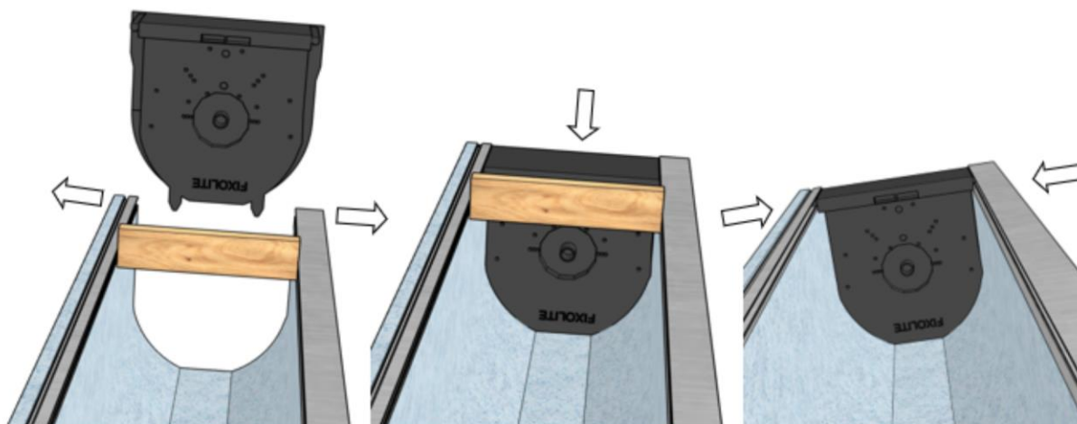
Figure 26 - Assemblage des joues sur le coffre
