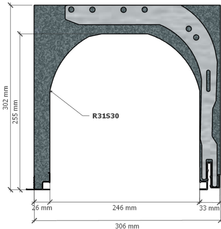
Coffre représenté : C-R31S30 8-28FR NG
