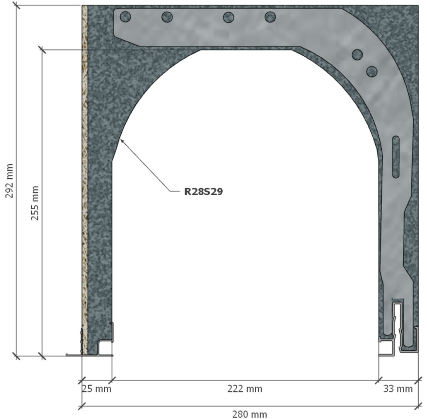
Coffre représenté : C-R28S29 8-28FR F-NG
