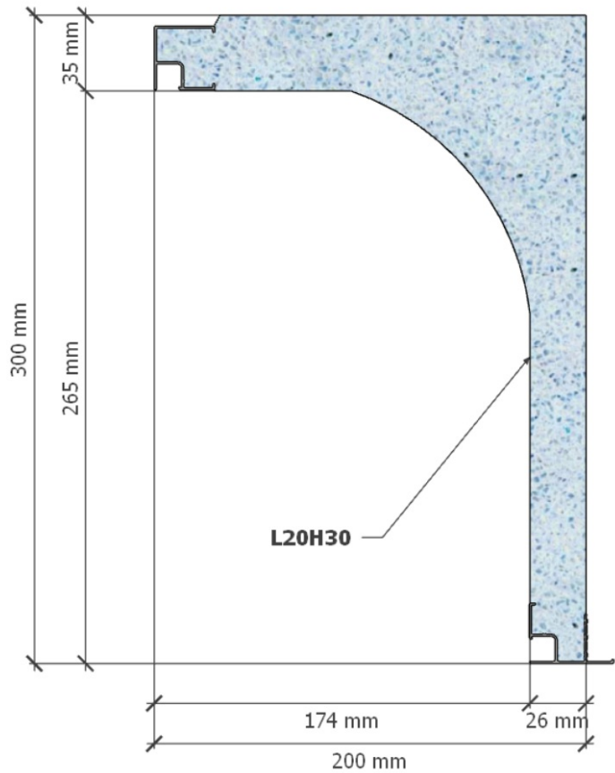
Coffre représenté : C-L20H30 8-8H
