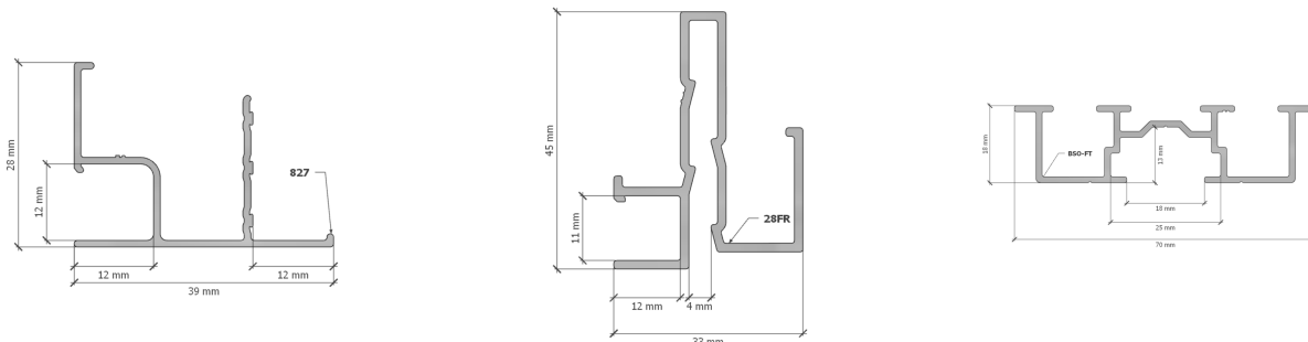
Coffre représenté : C-BSO28H32 8-FX-28FR TC-NG
