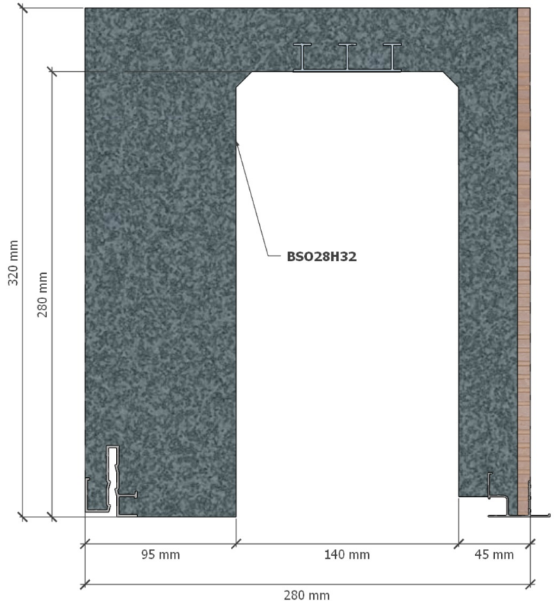
Coffre représenté : C-BSO28H32 8-FX-28FR TC-NG
