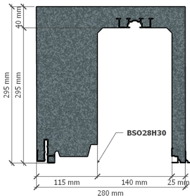
Coffre représenté : C-BSO28H30 8F-FT-28FR N
