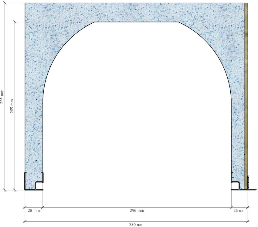
Coffre représenté : C-35H30 8-8H F
