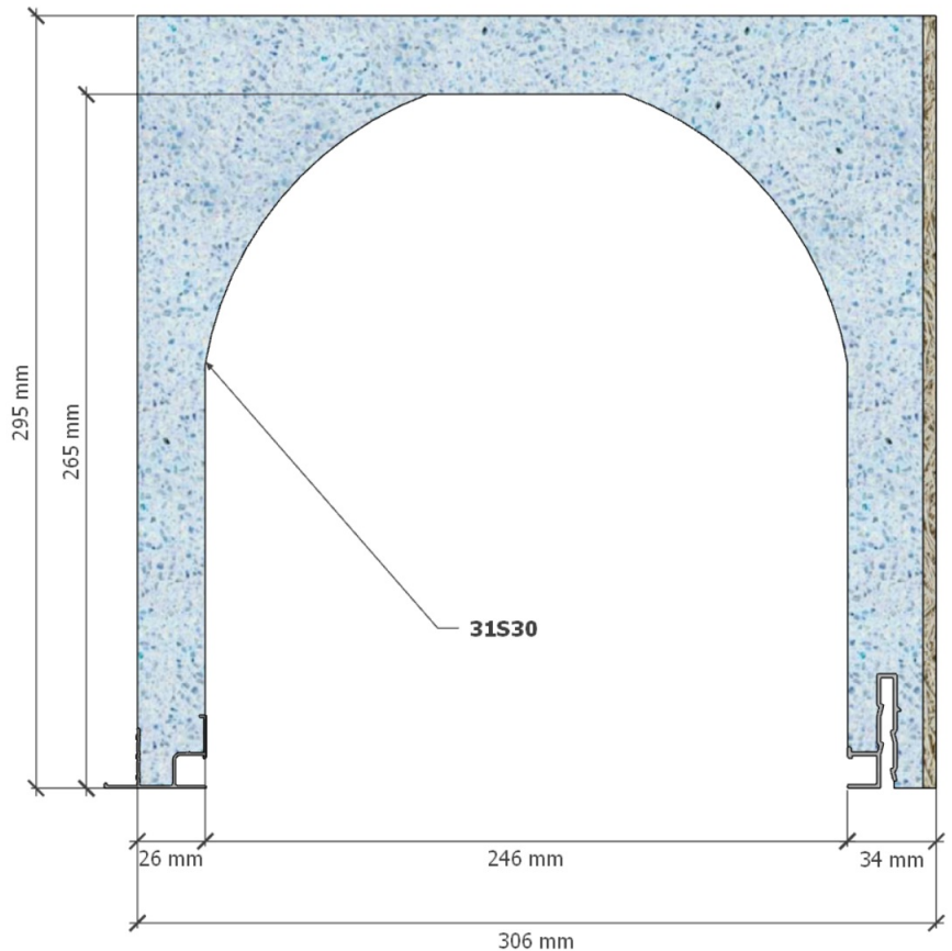
Coffre représenté : C-31S30 8-8R F-NB
