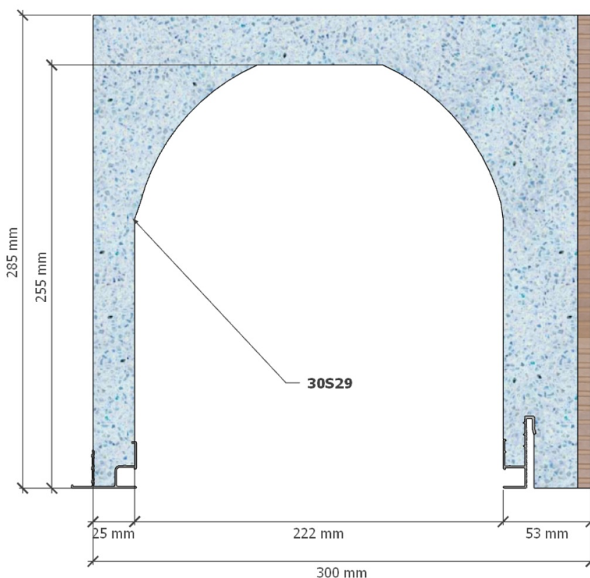
Coffre représenté : C-30S29 8-8E TC
