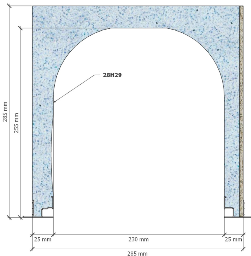
Coffre représenté : C-28H29 830-8 F
