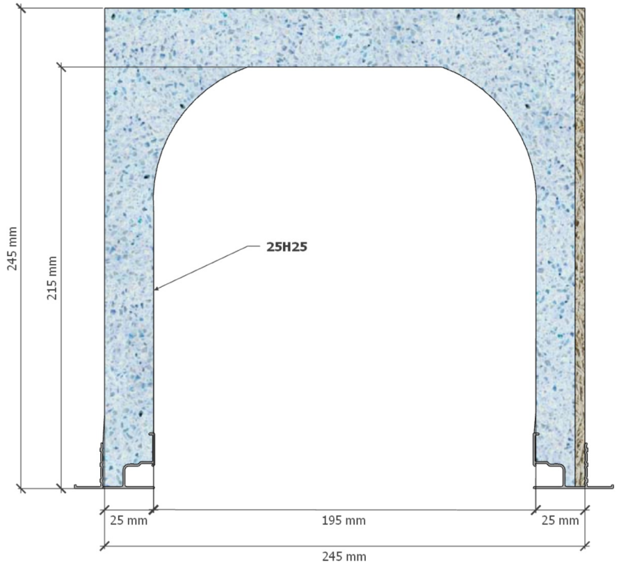
Coffre représenté : C-25H25 830-830 F
