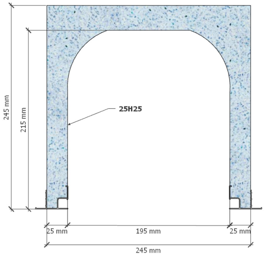
Coffre représenté : C-25H25 8-8
